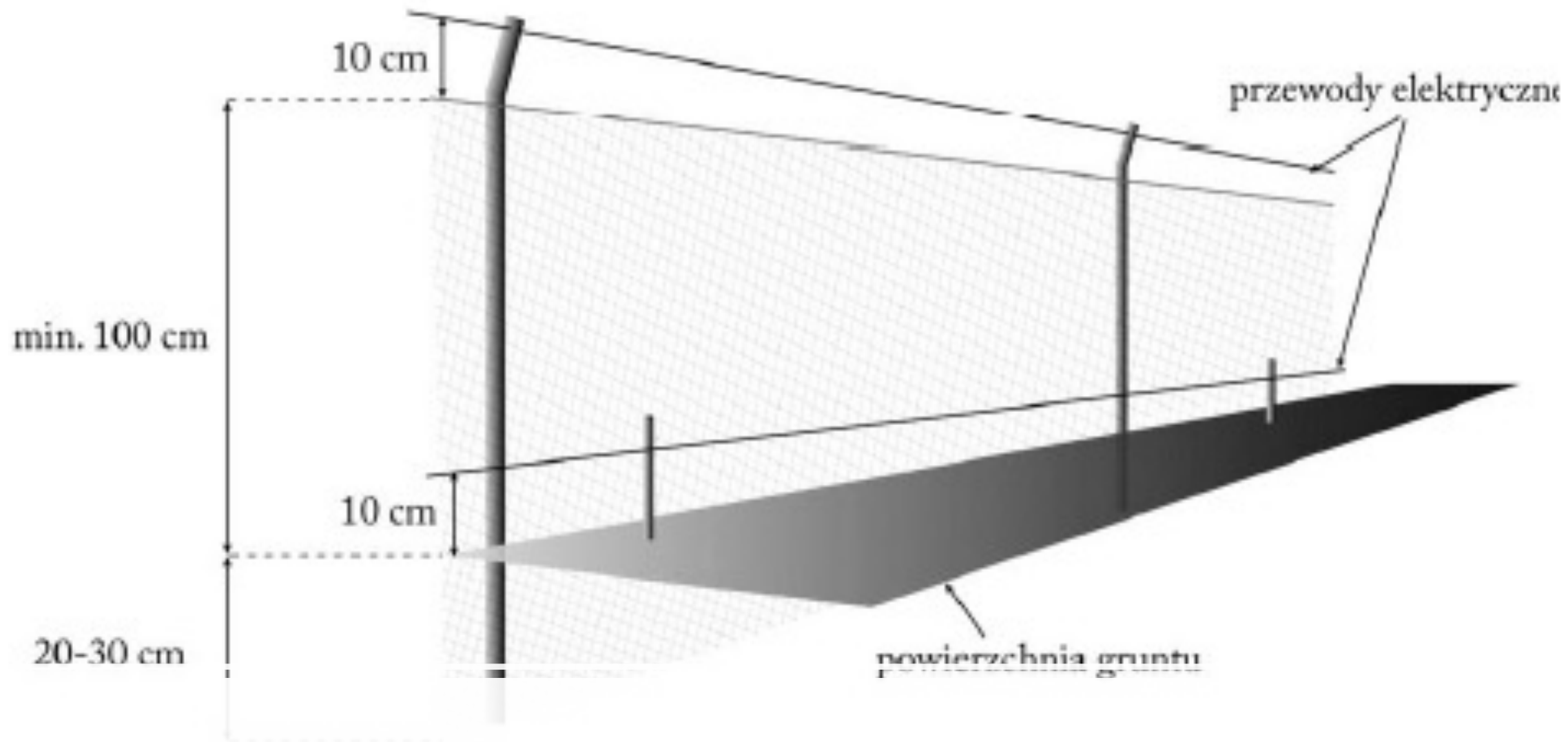
Modyfikacja z zastosowaniem przewodów elektrycznych
